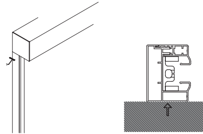
Dikme Önü Oluk Montaj (Alın Montaj) / Column Front Installation
