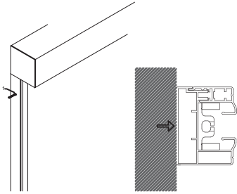
İki Dikme Arası Montaj / Installation Between Two Columns
