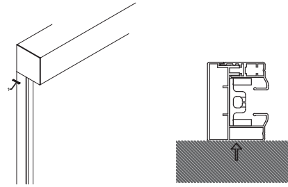
Dikme Önü Oluk Montaj (Alın Montaj) / Column Front Installation
